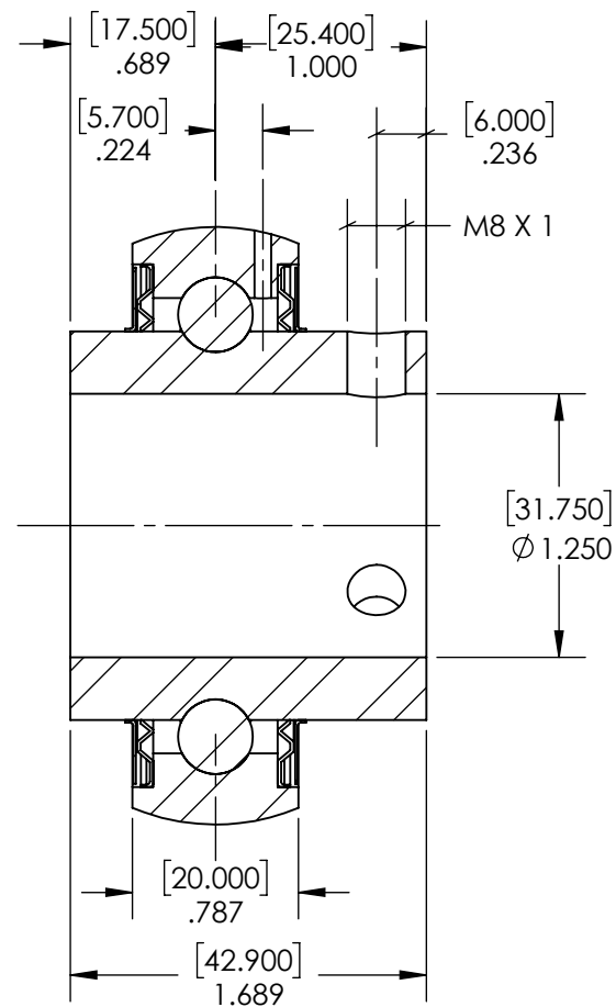
SECTION A-A
